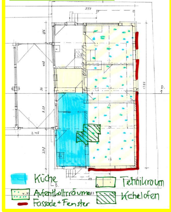
Pfadiheim Etappe 1 Wohnhausteil, EG (2019)
